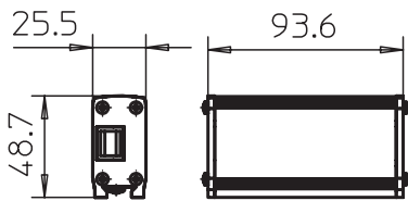
Abmessungen
