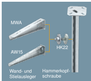
C21 Hängestiel Montage
