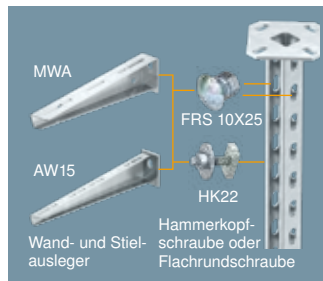
C41 Hängestiel Montage
