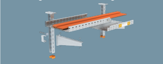
Befestigung US 5-System, für Funktionserhalt
