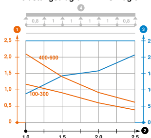
Belastungsdiagramm RKS-Magic®
